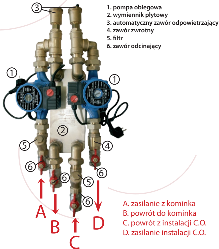
Rysunek 1. Schemat budowy zestawu mosiężnego wymiennikowo-plategowego.
